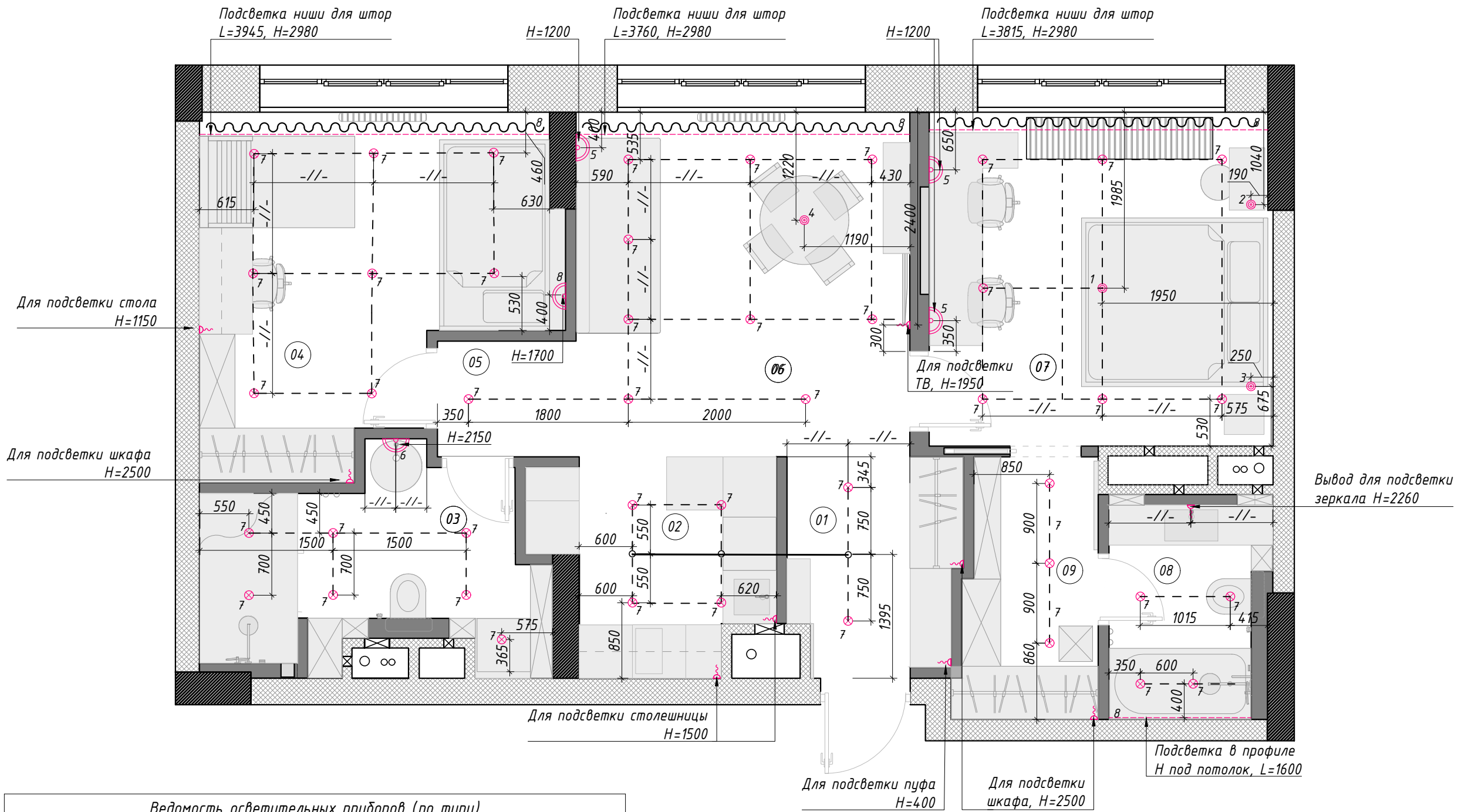
Ведомость осветительных приборов (по типу)
